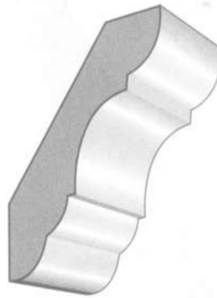
531 (MDF) 2-5/16
